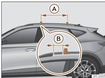
Fig. 194 Pontos de fixação das barras longitudinais para a bagageira do tejadilho.
