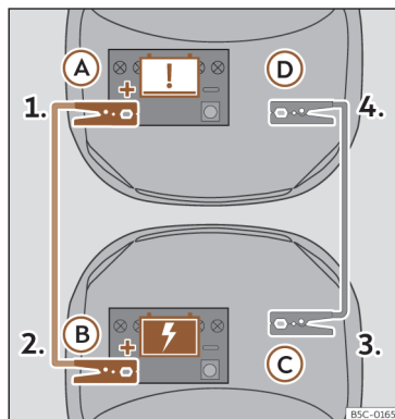
Fig. 207 Esquema de ligação para veículos com sistema Start-Stop.
