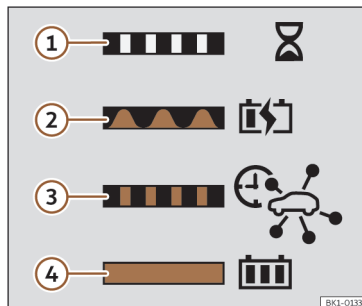
Fig. 63 Na face interior da tampa da tomada de carregamento da bateria: autocolante com informação sobre o indicador do processo de carregamento.
