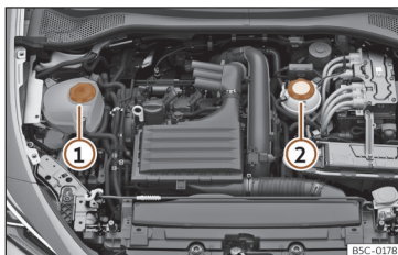
Fig. 217 Compartimento do motor: Depósitos do líquido de refrigeração
