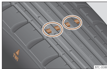
Fig. 231 Perfil do pneu: indicadores de desgaste.
