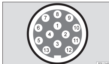
Fig. 202 Representação esquemática: atribuição dos pinos da tomada de corrente para reboque.
