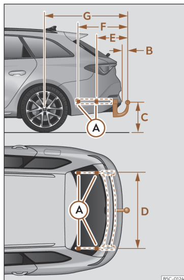
Fig. 206 Quotas e pontos de fixação para a montagem posterior de um dispositivo de reboque.
