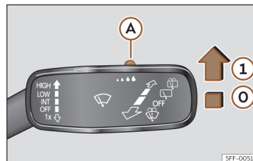
Fig. 82 Manípulo do limpa-vidros: ajustar o sensor de chuva (A).
