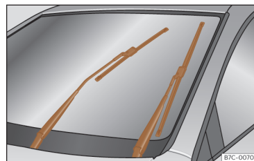
Fig. 183 Limpa-vidros em posição de serviço.
