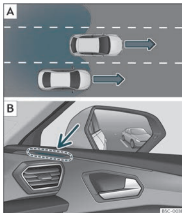
Fig. 171 Esquema: [A] Situação numa ultrapassagem na faixa de rodagem central e incorporação posterior na faixa de rodagem direita. [B] Indicação do assistente de mudança de faixa na luz de controlo do lado direito.
