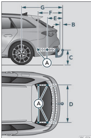
Fig. 188 Quotas e pontos de fixação para a montagem posterior de um dispositivo de reboque.
