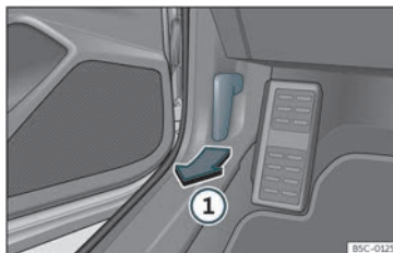
Fig. 201 Alavanca de desbloqueio no espaço para a zona dos pés do condutor.
