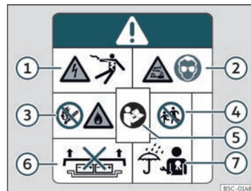
Fig. 190 Rótulo de advertência da bateria de alta tensão.
