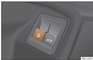
Fig. 212 Porta do condutor: desbloqueio da tampa do depósito
