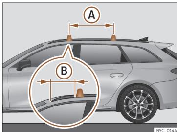
Fig. 137 Pontos de fixação das barras longitudinais para a bagageira do tejadilho (Leon Sportstourer).
