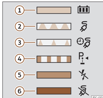
Fig. 207 Na parte interior da tampa da tomada de carregamento da bateria: autocolante com informação sobre o indicador do processo de carregamento.
