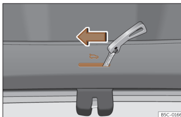
Fig. 90 Pormenor da bagageira: destrancagem de emergência (Leon).
