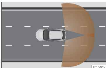
Fig. 164 Zonas de deteção dos sensores
