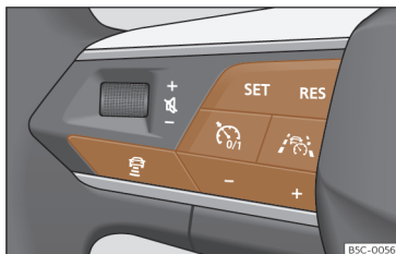
Fig. 179 Lado esquerdo do volante multifunções: botões para a utilização do Travel Assist.
