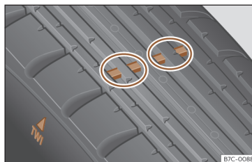
Fig. 238 Perfil do pneu: indicadores de desgaste.
