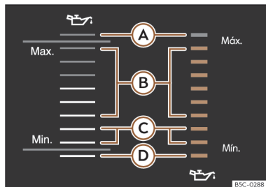
Fig. 232 No ecrã do sistema de infotainment: possíveis visualizações do indicador do nível do óleo do motor.
