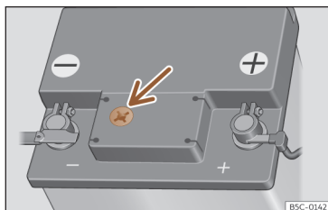
Fig. 226 Janela de inspeção na parte superior da bateria de 12 volts (representação esquemática).
