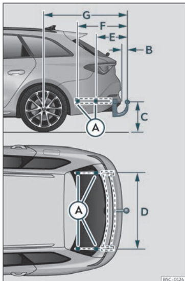
Fig. 199 Quotas e pontos de fixação para a montagem posterior de um dispositivo de reboque.
