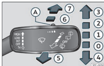
Fig. 99 Utilização do limpa-para-brisas e do limpa-vidros traseiro.
