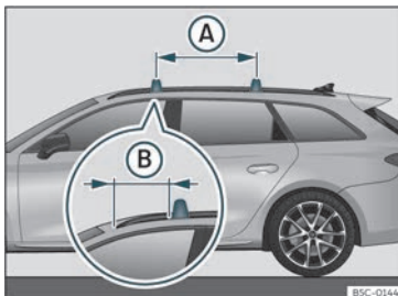
Fig. 136 Pontos de fixação das barras longitudinais para a bagageira do tejadilho (Leon Sportstourer).
