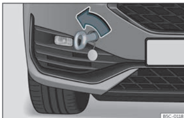
Fig. 48 Parte direita do para-choques dianteiro: argola de reboque enroscada.
