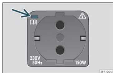
Fig. 141 Na bagageira: tomada de corrente de 230 Volts.
