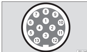
Fig. 197 Esquema: atribuição dos pinos da tomada de corrente para reboque.
