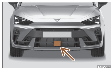
Fig. 130 No para-choques dianteiro: sensor de radar.
