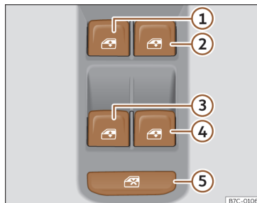
Fig. 88 Pormenor da porta do condutor: comandos das janelas.
