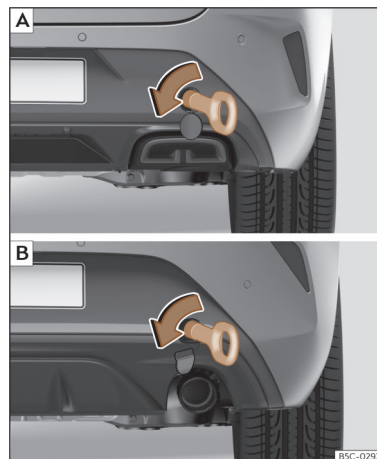
Fig. 222 No lado direito do para-choques traseiro: argola de reboque enroscada. [A] Leon Sportstourer; [B] Leon.
