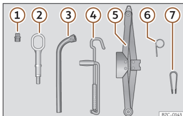
Fig. 213 Na bagageira, debaixo da cobertura da superfície de carga: ferramentas de bordo.
