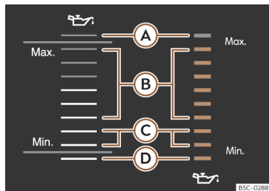
Fig. 236 No ecrã do sistema de infotainment: possíveis visualizações do indicador do nível do óleo do motor.
