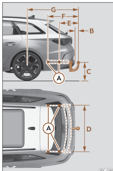
Fig. 208 Quotas e pontos de fixação para a montagem posterior de um dispositivo de reboque.
