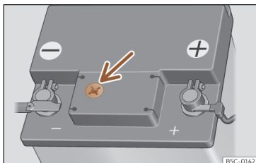
Fig. 239 Janela de inspeção na parte superior da bateria de 12 volts (representação esquemática).
