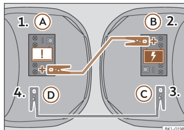
Fig. 216 Esquema de ligação dos cabos de emergência.
