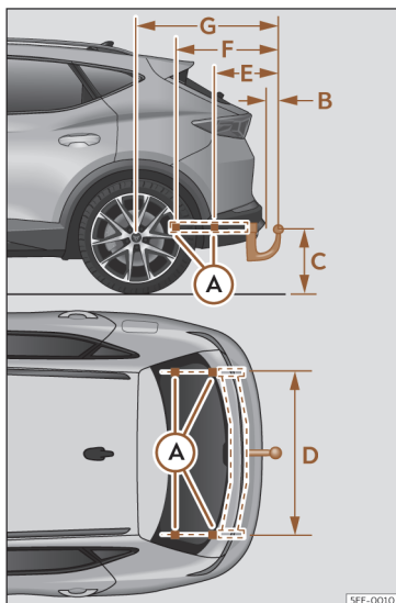
Fig. 200 Quotas e pontos de fixação para a montagem posterior de um dispositivo de reboque.
