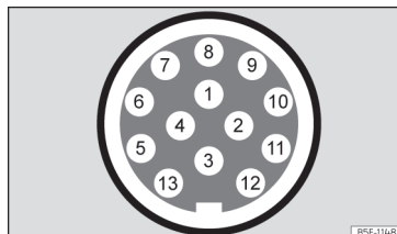
Fig. 196 Representação esquemática: atribuição dos pinos da tomada de corrente para reboque.
