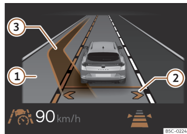
Fig. 149 No ecrã do painel de instrumentos: visualização da mudança de faixa de rodagem assistida (representação esquemática).
