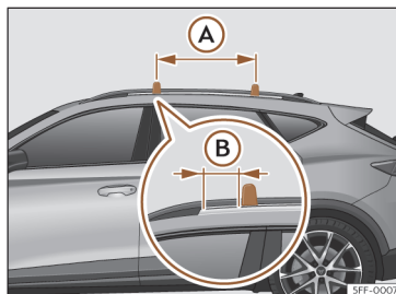
Fig. 195 Pontos de fixação das barras longitudinais para a bagageira do tejadilho.
