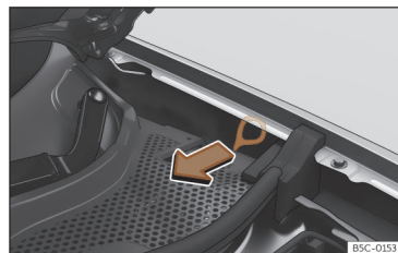
Fig. 63 Entre a lateral esquerda e a dobradiça do capô do motor Puxador para o desbloqueio manual de emergência do conector de carregamento.
