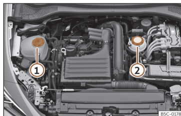
Fig. 218 Compartimento do motor: Depósitos do líquido de refrigeração
