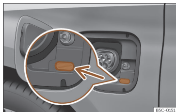
Fig. 61 Por trás da tampa da tomada de carregamento da bateria: indicador do processo de carregamento.
