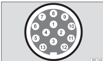
Fig. 187 Esquema: atribuição dos pinos da tomada de corrente para reboque.
