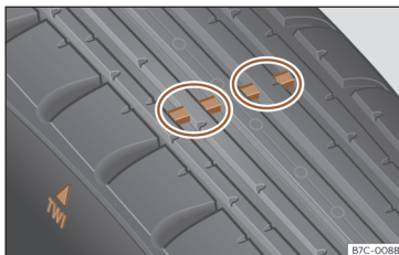
Fig. 205 Perfil do pneu: indicadores de desgaste.
