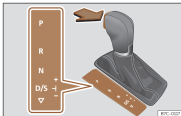
Fig. 137 Bloqueio da alavanca seletora.
