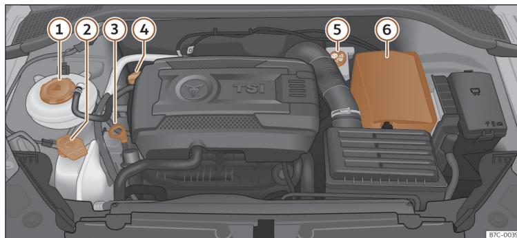
Fig. 194 Figura orientadora da posição dos elementos.
