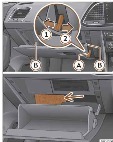
Fig. 46 Porta-luvas (volante à direita): acesso à caixa de fusíveis.
