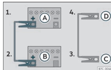
Fig. 40 Esquema de ligação para veículos com sistema Start-Stop.
