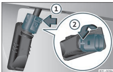
Fig. 54 Luz da matrícula: desmontar o porta-lâmpadas.
