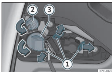
Fig. 52 desmontar o porta-lâmpadas.
