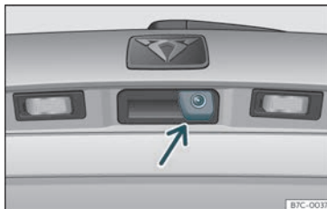
Fig. 153 No manípulo da porta da bagageira: câmara de visão periférica.
