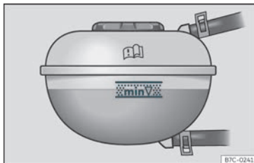
Fig. 204 No compartimento do motor: marca no depósito de expansão do líquido de refrigeração.
