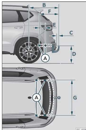
Fig. 196 Quotas e pontos de fixação para a montagem posterior de um dispositivo de reboque.
