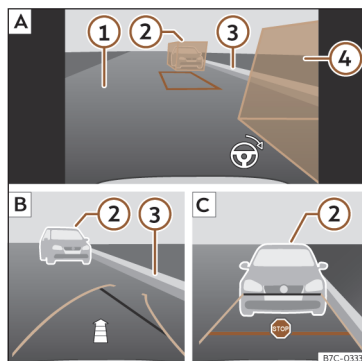
Fig. 138 Visualização no ecrã do sistema de infotainment: assistente de marcha-atrás, modo 2.
