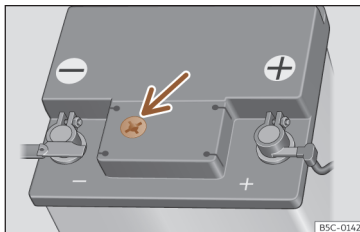
Fig. 202 Janela de inspeção na parte superior da bateria de 12 volts (representação esquemática).
