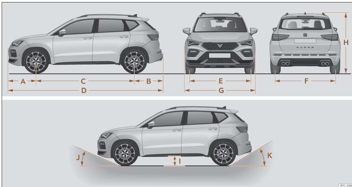
Fig. 218 Dimensões
