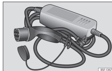
Fig. 69 Cabo de carregamento para tomadas de corrente.
