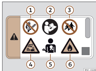
Fig. 234 Bateria de 48 volts: advertência de perigos
