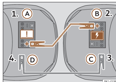
Fig. 210 Esquema de ligação dos cabos de emergência.
