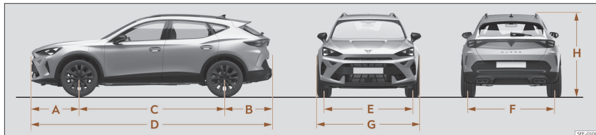
Fig. 251 Dimensões
