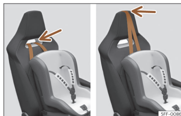
Fig. 47 Banco do passageiro: ajuste e montagem em função do cinto Top Tether.
