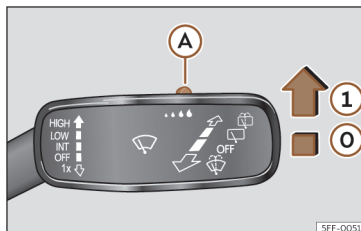
Fig. 112 Manípulo do limpa-vidros: ajustar o sensor de chuva A .
