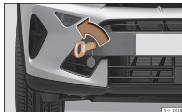
Fig. 214 Parte direita do para-choques dianteiro: argola de reboque enroscada.
