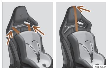
Fig. 48 Banco do passageiro: ajuste e montagem em função do cinto Top Tether.
