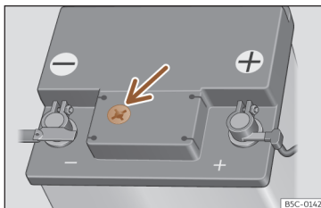
Fig. 201 Janela de inspeção na parte superior da bateria de 12 volts (representação esquemática).
