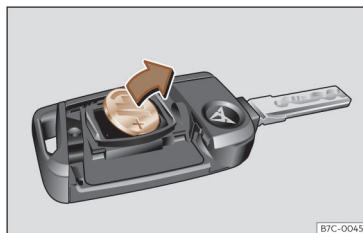
Fig. 45 Chave do veículo: remoção da pilha.
