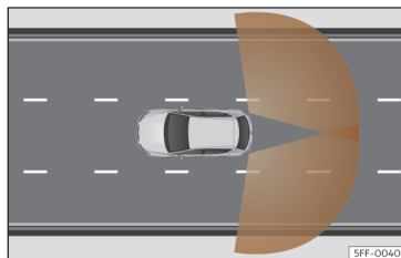
Fig. 105 Zonas de deteção dos sensores.
