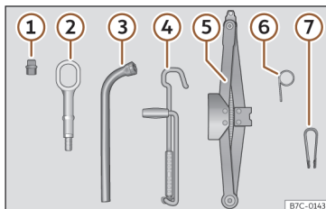
Fig. 178 Na bagageira, debaixo da cobertura da superfície de carga: ferramentas de bordo.
