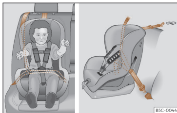
Fig. 39 Nos bancos traseiros: montagens da cadeira para crianças.
