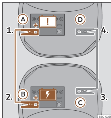
Fig. 182 Esquema de ligação para veículos com sistema Start-Stop.
