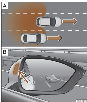
Fig. 123 Esquema: A Ultrapassagem na faixa de rodagem central e incorporação posterior na faixa de rodagem direita. B Indicação do assistente de mudança de faixa no lado direito.
