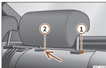
Fig. 73 Encostos de cabeça traseiros desmontagem.
