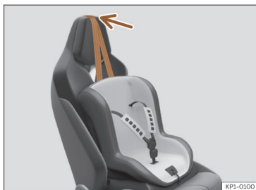
Fig. 46 Banco do passageiro: ajuste e montagem em função do cinto Top Tether.
