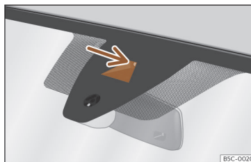
Fig. 125 No para-brisas: área de campo visual do sistema de aviso de saída da faixa de rodagem.
