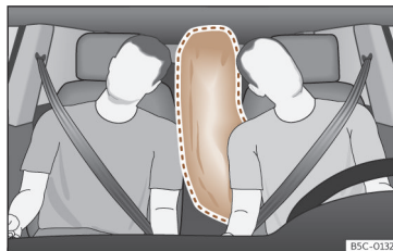
Fig. 33 Airbag central ativado totalmente (raio de alcance).
