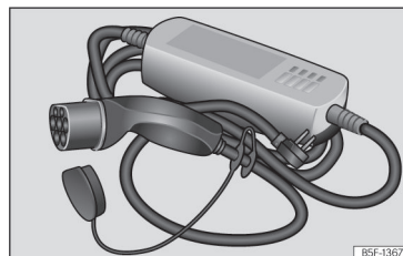
Fig. 66 Cabo de carregamento para tomadas de corrente.
