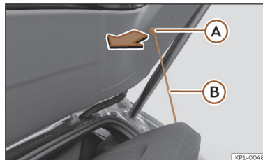
Fig. 181 Na bagageira: desmontar e montar a chapeleira.
