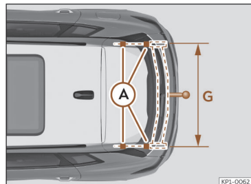
Fig. 200 Dispositivo de reboque: cotas e pontos de fixação.
