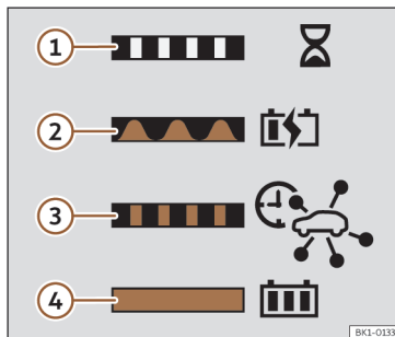
Fig. 62 Na face interior da tampa da tomada de carregamento da bateria: autocolante com informação sobre o indicador do processo de carregamento.
