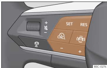
Fig. 130 No volante multifunções: botões para utilizar o limitador de velocidade.
