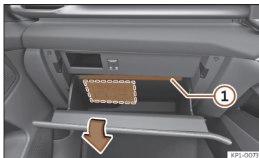
Fig. 216 Veículos com volante à direita: caixa de fusíveis por trás do porta-luvas, no lado do passageiro.
