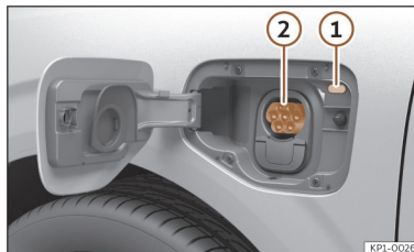
Fig. 58 Por trás da tampa de carregamento da bateria na parte dianteira esquerda: tomada de carregamento.
