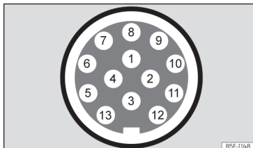
Fig. 195 Representação esquemática: atribuição dos pinos da tomada de corrente para reboque.
