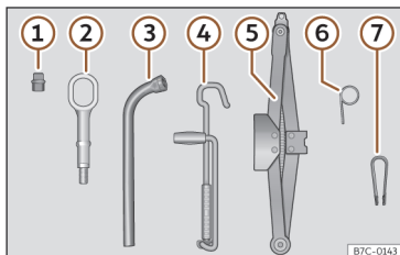
Fig. 202 Na bagageira, debaixo da cobertura da superfície de carga: ferramentas de bordo.
