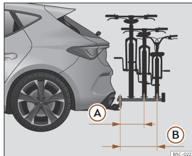
Fig. 197 Representação esquemática da saliência máxima da carga num porta-bicicletas para duas ou três bicicletas.
