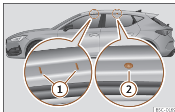
Fig. 193 Pontos de fixação das barras longitudinais para a bagageira do tejadilho (Leon).
