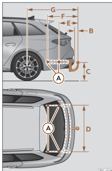
Fig. 198 Quotas e pontos de fixação para a montagem posterior de um dispositivo de reboque.
