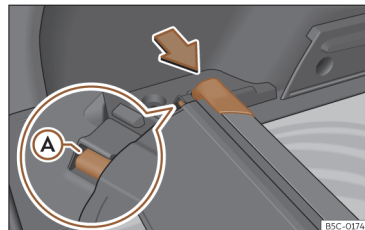
Fig. 178 Na bagageira: alojamento para guardar a chapeleira.
