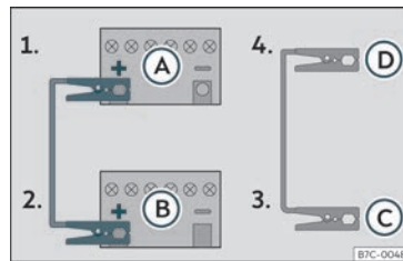
Fig. 42 Esquema de ligação para veículos com sistema Start-Stop.
