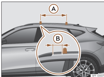
Fig. 185 Pontos de fixação das barras longitudinais para a bagageira do tejadilho.
