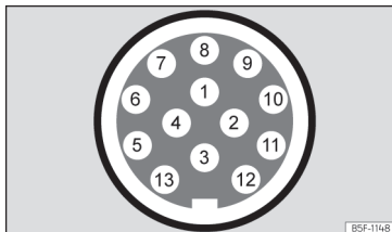
Fig. 186 Representação esquemática: atribuição dos pinos da tomada de corrente para reboque.
