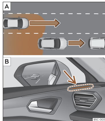
Fig. 144 Esquema: [A] Ultrapassagem com trânsito na parte traseira. [B] Indicação do assistente de mudança de faixa no lado esquerdo.
