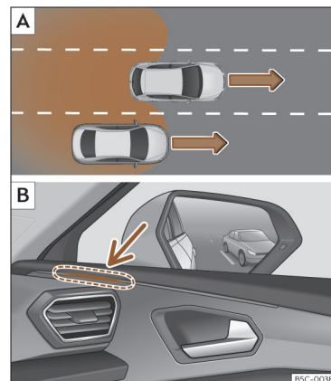
Fig. 145 Esquema: [A] Ultrapassagem na faixa de rodagem central e incorporação posterior na faixa de rodagem direita. [B] Indicação do assistente de mudança de faixa no lado direito.
