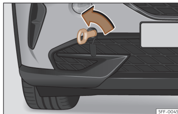
Fig. 200 Parte direita do para-choques dianteiro: argola de reboque enroscada.
