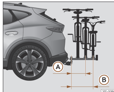
Fig. 189 Representação esquemática da saliência máxima da carga num porta-bicicletas para duas ou três bicicletas.
