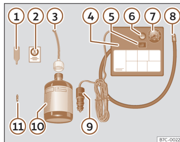
Fig. 230 Representação standard: conteúdo do kit antifuros.
