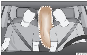
Fig. 32 Airbag central ativado totalmente (raio de alcance).
