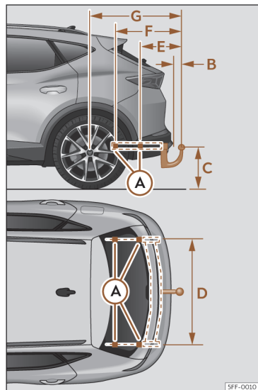
Fig. 190 Quotas e pontos de fixação para a montagem posterior de um dispositivo de reboque.
